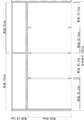
側面
